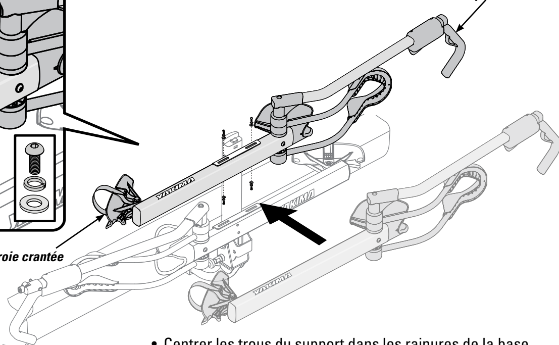
Bras pivotant
